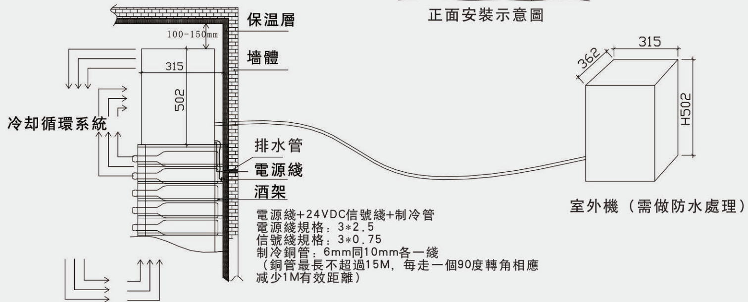
安裝剖面圖
