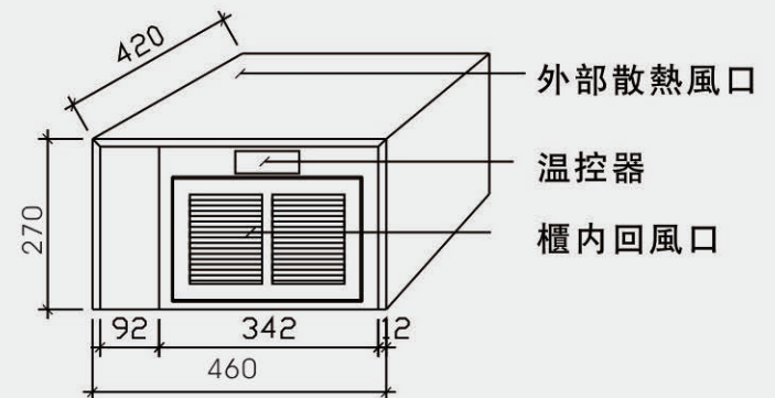
正面圖
