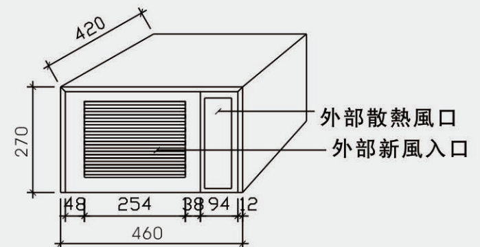
背面圖
