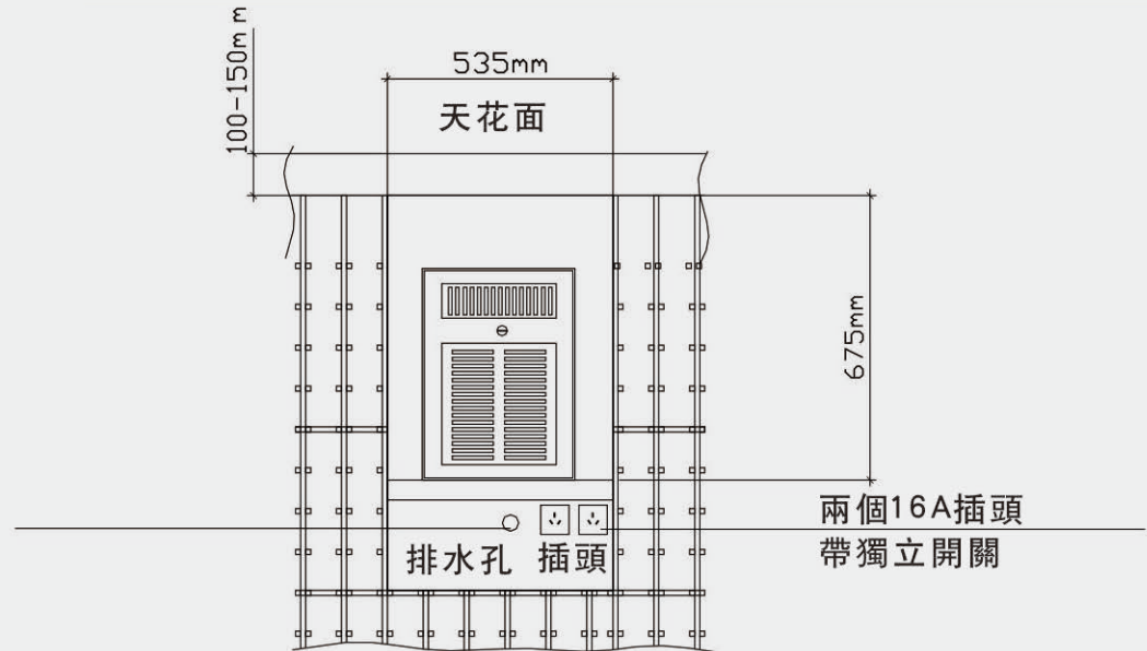
正面安裝示意圖
